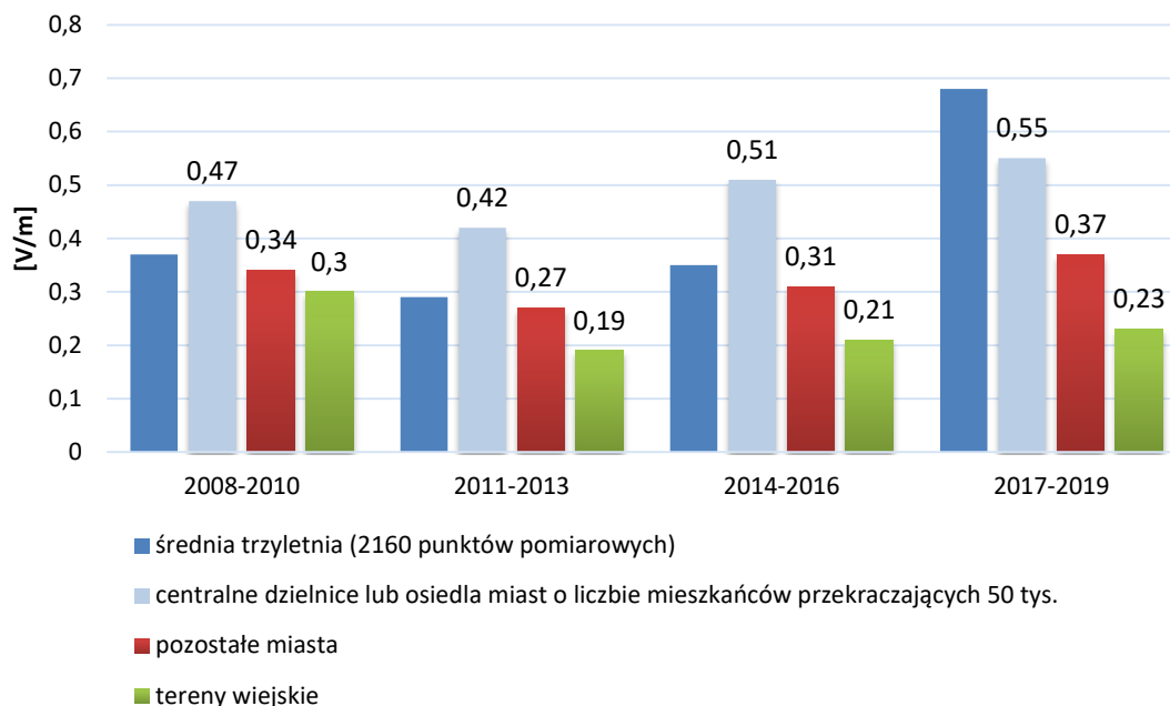
Rysunek 48. Zmiana średniego natężenia składowej elektrycznej uzyskanej na poszczególnych obszarach w tych samych lokalizacjach w kolejnych cyklach pomiarowych 142
